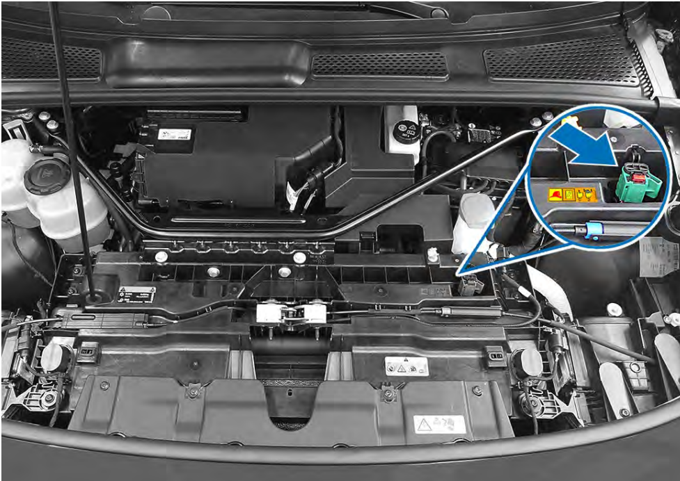
Trennstelle im Vorderwagen Elektroauto (ID.3), siehe auch Neue Kennzeichnung ab ID.7 .
