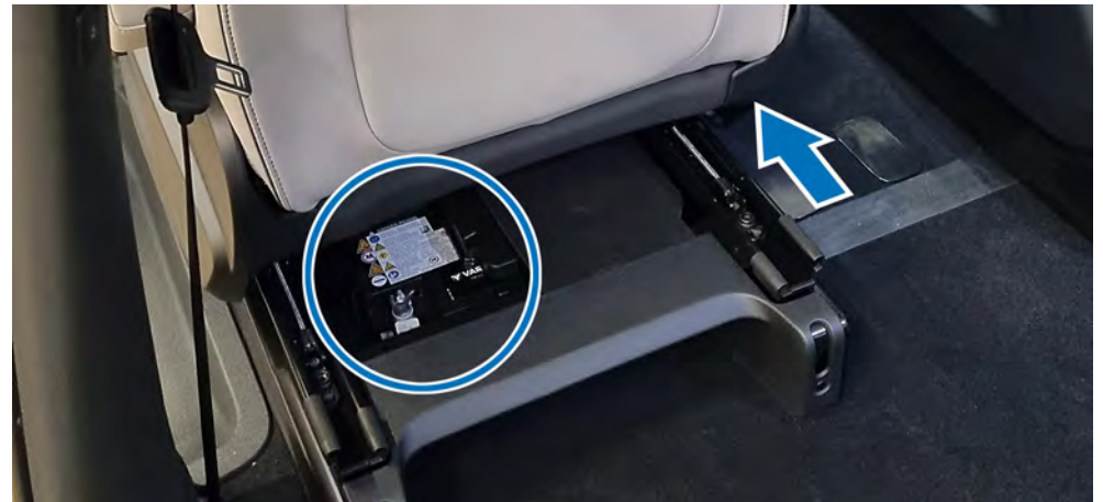
Einbauort im Fahrgastraum unter Fahrersitz (Beispiel ID. BUZZ).
