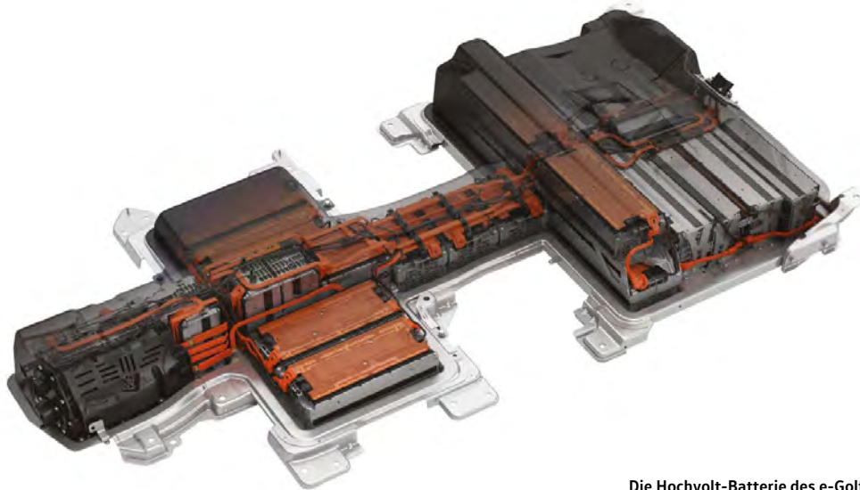
Die Hochvolt-Batterie des e-Golf
