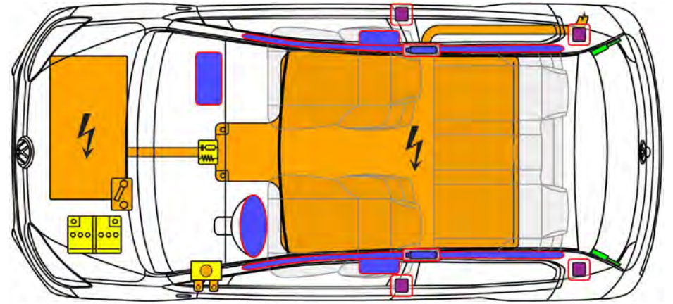
Einbauort der Hochvolt-Batterie im e-up!
