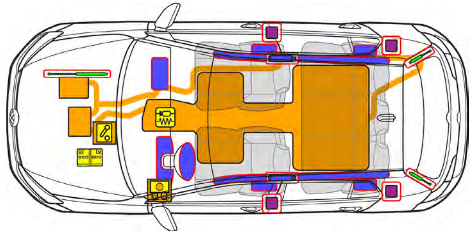
Einbauort der Hochvolt-Batterie im e-Golf.
