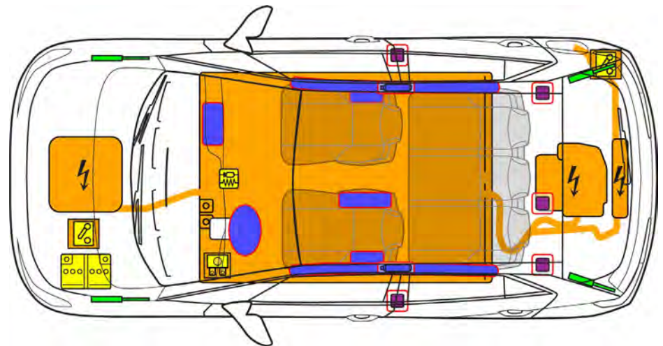
Einbauort der Hochvolt-Batterie im ID.3
