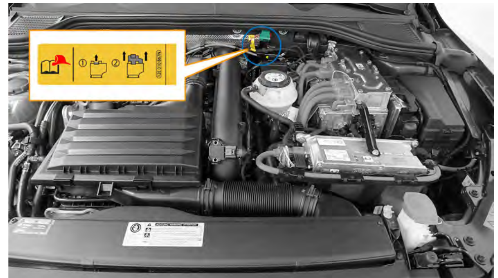
Trennstelle im Vorderwagen Hybridfahrzeuge (Golf GTE ab 2020), siehe auch Neue Kennzeichnung ab ID.7.
