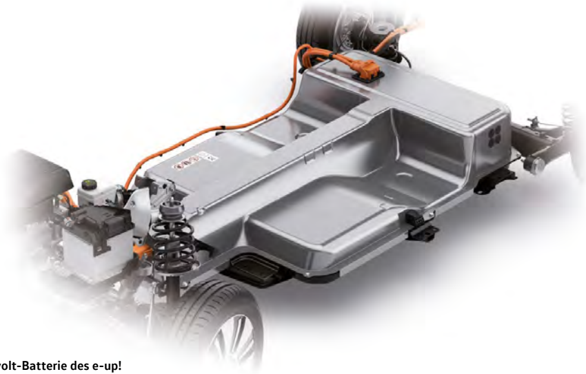
Die Hochvolt-Batterie des e-up!
