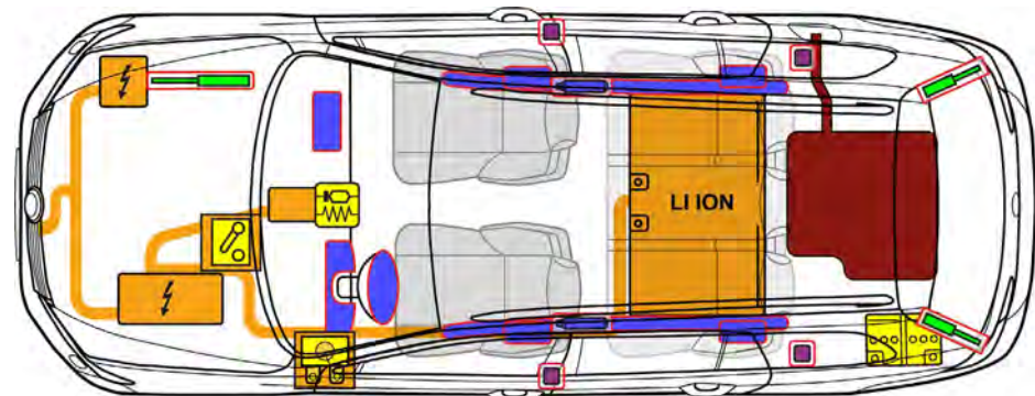
Einbauort der Hochvolt-Batterie im Passat GTE.
