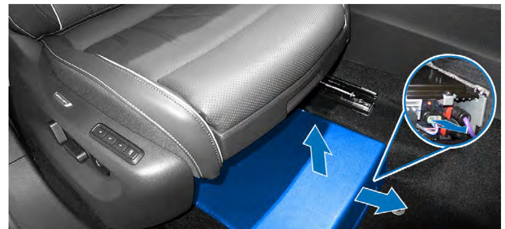
Abklemmen des 48-Volt-Bordnetzes beim Tiguan ab 2023.
