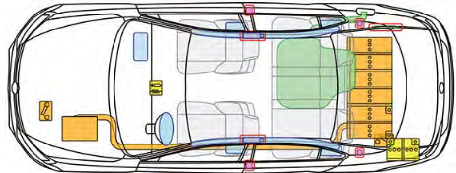
Einbauort der Hochvolt-Batterie im Jetta Hybrid. (Die Illustration entspricht nicht der aktuellen ISO 17840.)
