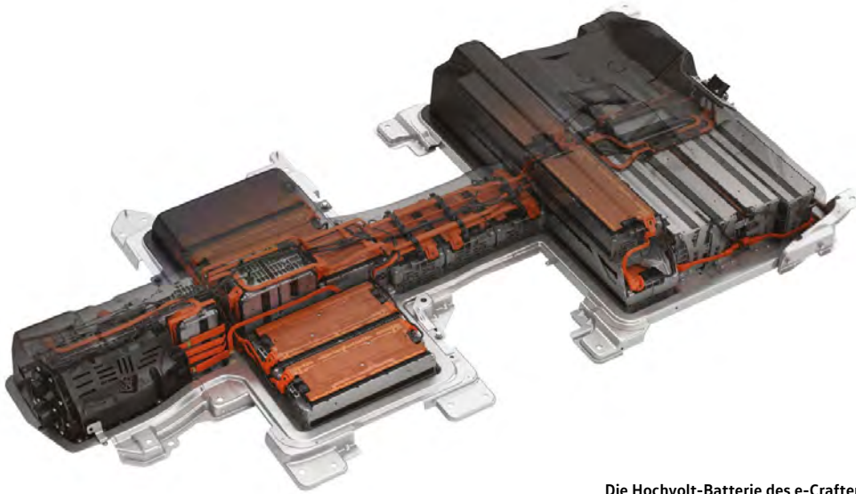
Die Hochvolt-Batterie des e-Crafter
