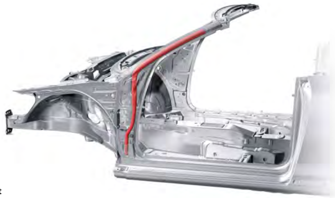
A-Säulen-Verstärkung beim Cabriolet
