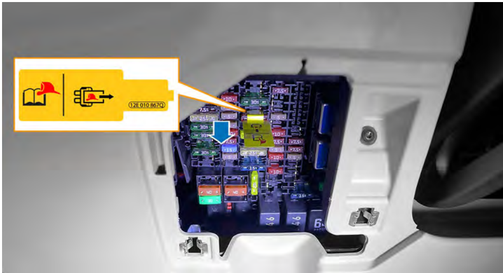
Trennstelle im Fahrgastraum, Armaturentafel am Sicherungsträger, siehe auch Neue Kennzeichnung ab ID.7.
