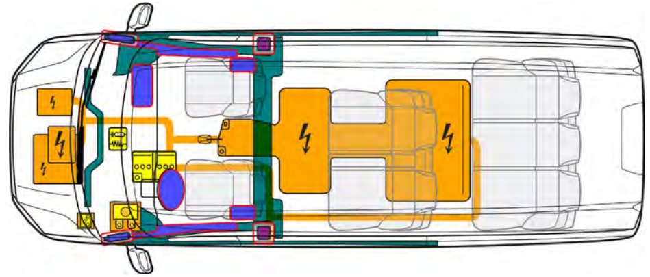
Einbauort der Hochvolt-Batterie im e-Crafter
